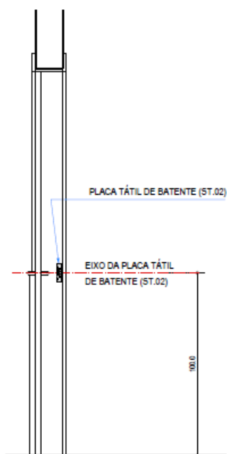
POSICIONAMENTO DE PLACA TÁTIL DE BATENTE (ST.02) DIMENSÕES EM CENTÍMETROS
