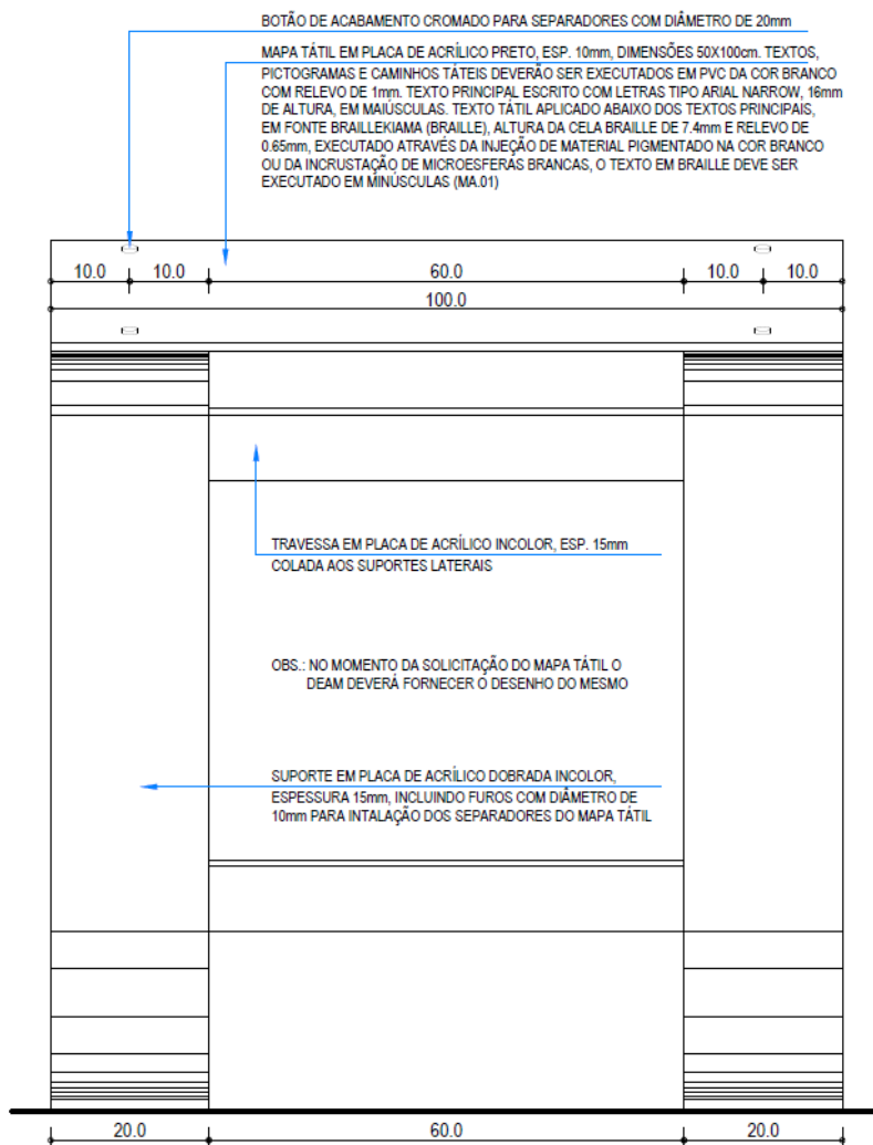
MA.01 - MAPA TÁTIL E MA.02 - SUPORTE PARA MAPA TÁTIL VISTA FRONTAL
