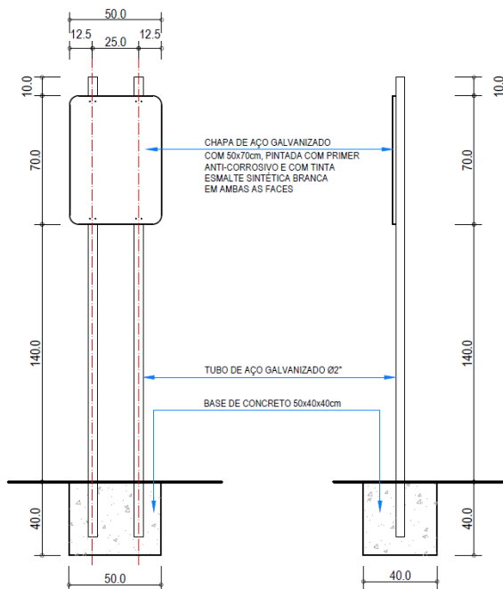
SV.06 - SUPORTE PARA SINALIZAÇÃO VERTICAL VISTA FRONTAL E VISTA LATERAL
