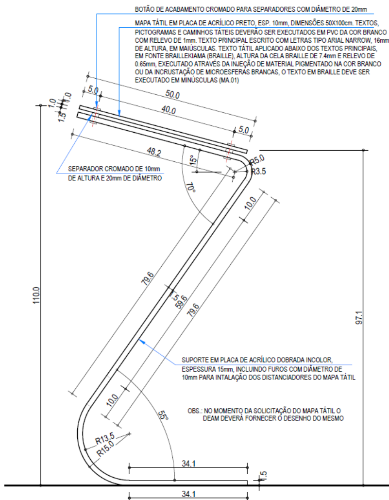
MA.01 - MAPA TÁTIL E MA.02 - SUPORTE PARA MAPA TÁTIL VISTA LATERAL
