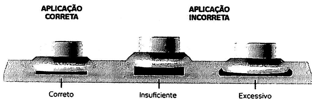
Figura 01 – detalhe do aperto correto
