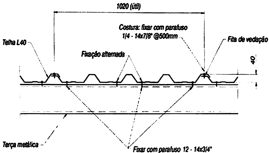
Figura 02 – Detalhe da fixação
